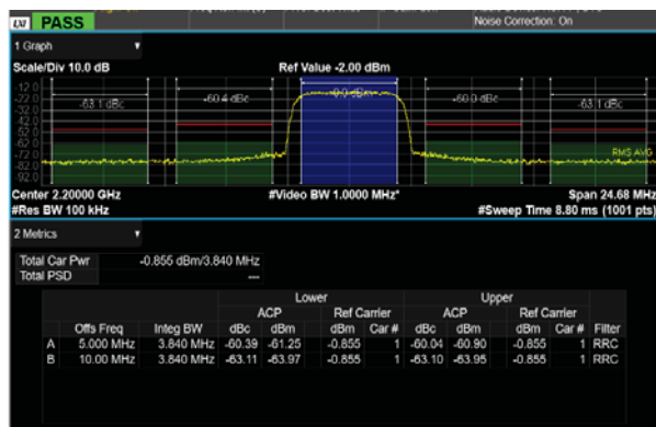
3GPP WCDMA TM1 - 64DPCH ACPR
